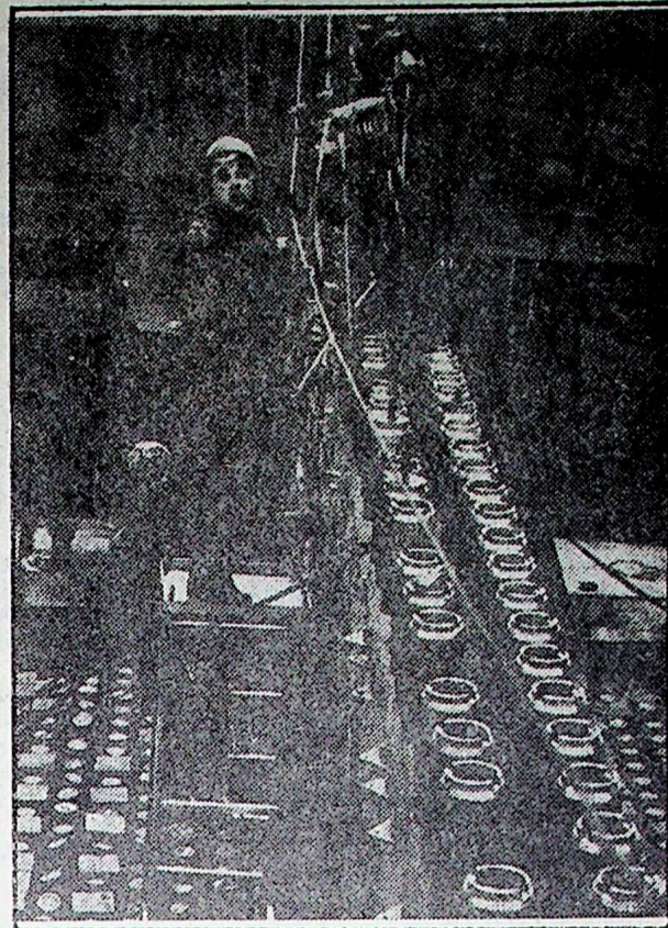
Ноябрь 1982 года. Нарастывание и сварка трактов реактора бригадой Г.Куракина.
